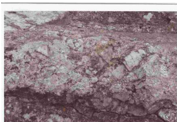
Pegmatites. Sainte-Barbe
